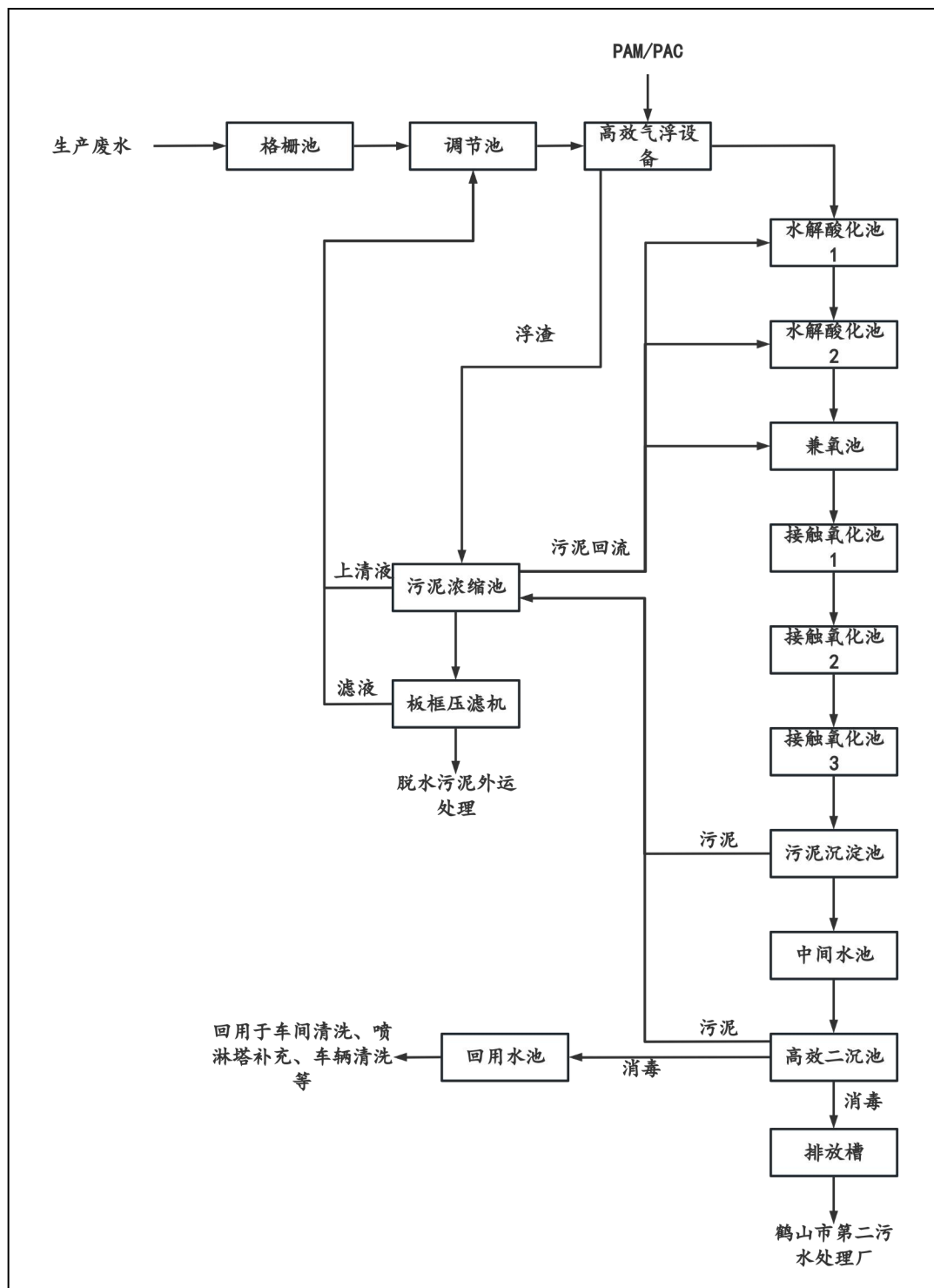
图 8.1-1 本项目生产废水处理站工艺流程图
