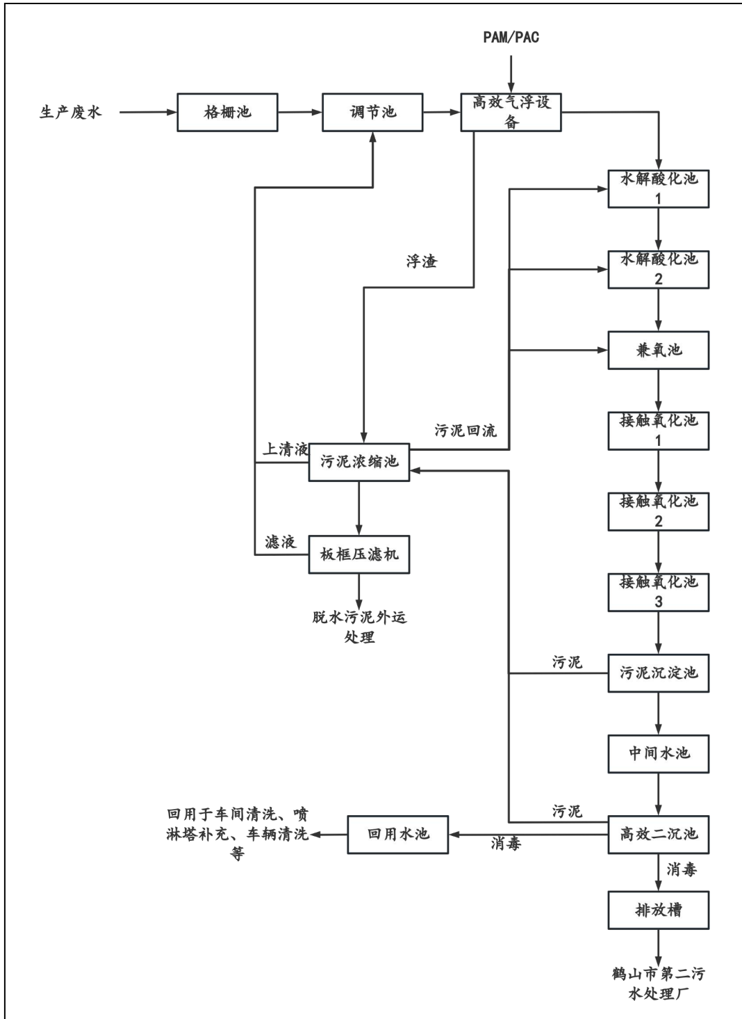
图 6.1-1 本项目污水处理站工艺流程图
