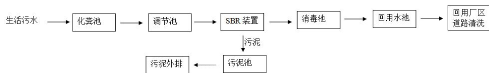
图4-2 污水处理工艺流程图
