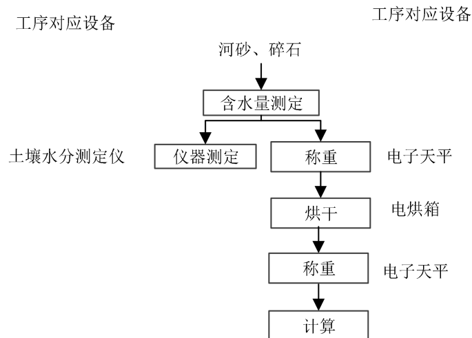
图2-13 砂石含水量测定流程图
