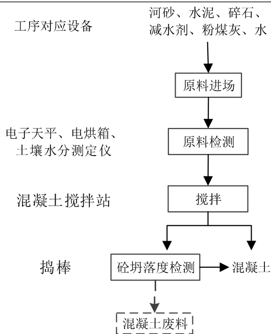
图2-10 混凝土生产工艺流程图
