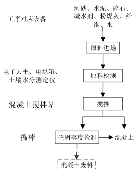
图2-7 混凝土生产工艺流程图
