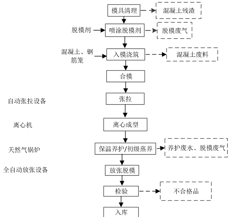
图2-5 管桩生产工艺流程图
