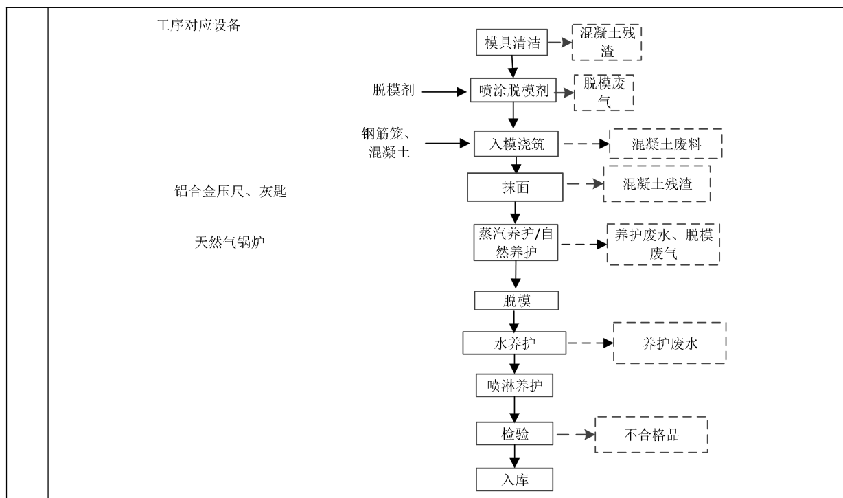
图2-8 管片生产工艺流程图
