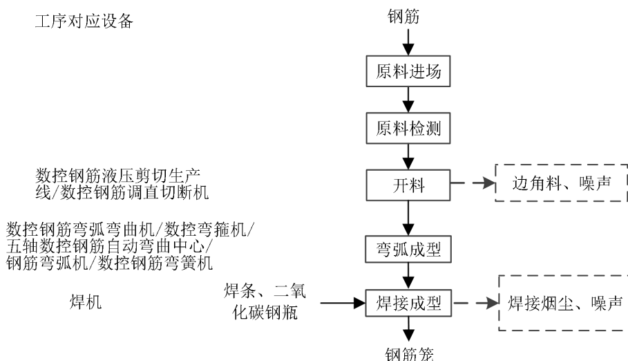
图2-6 钢筋笼生产工艺流程图
