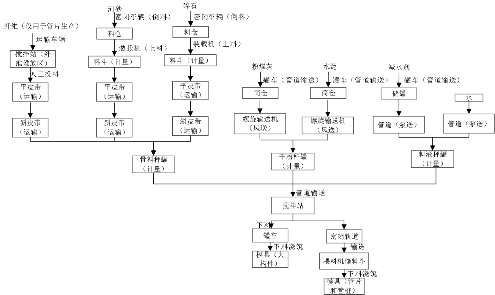
图 4-1 混凝土生产的设备流程图
