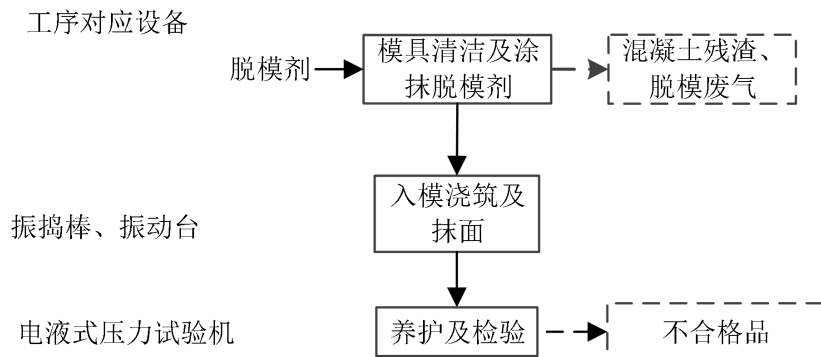
图2-12 试块制作工艺流程图
