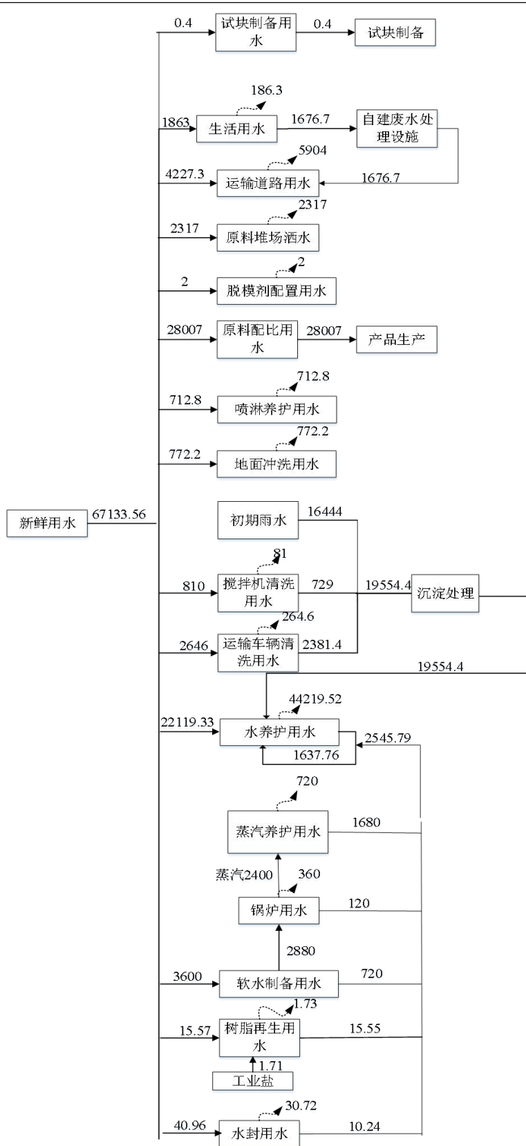
图2-1 项目水平衡图 (单位: m^3/a )
