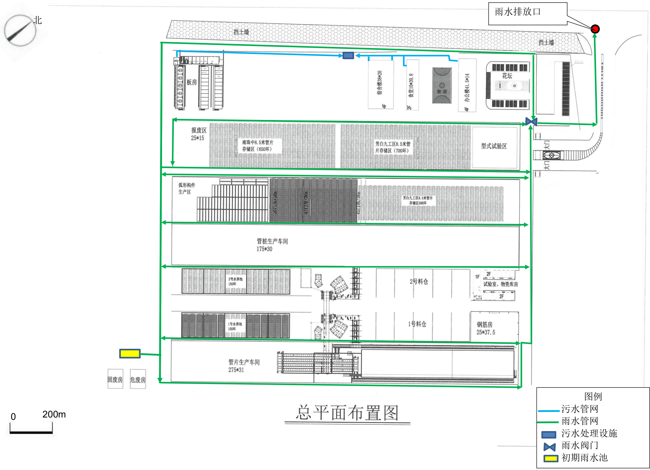
附图4 雨污管网图
