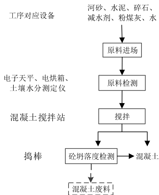
图2-4 混凝土生产工艺流程图
