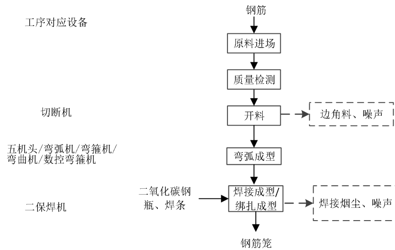
图 2-9 钢筋笼生产工艺流程图
