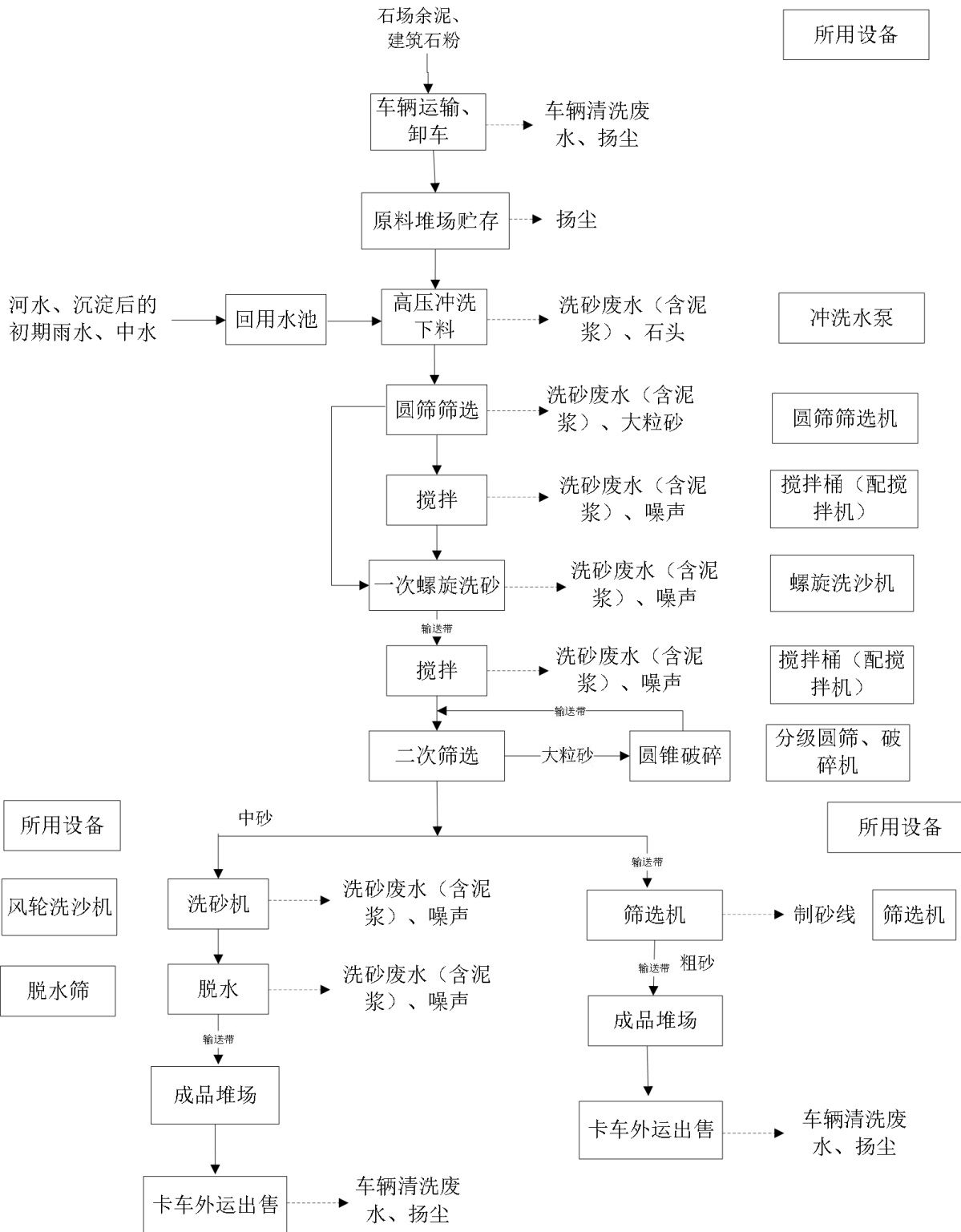
图 2-2 洗砂线生产工艺流程及排污节点图
