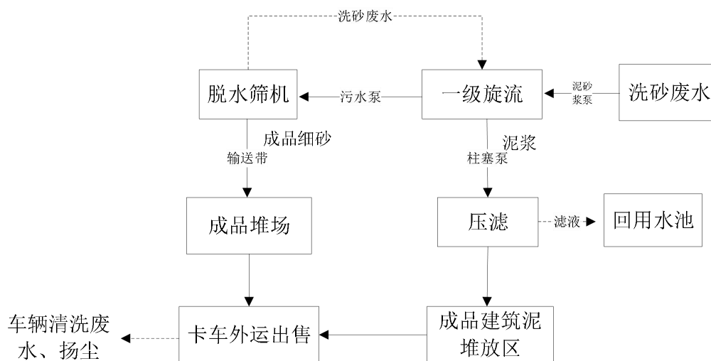
图 2-4 洗砂废水（含泥浆）处理流程
