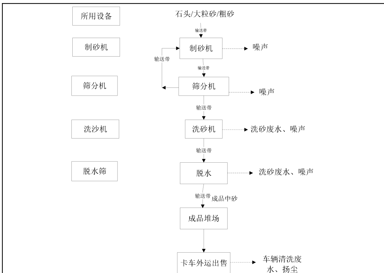
图 2-3 制砂线生产工艺流程及排污节点图
