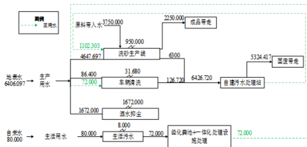
图2-2项目旱季全厂水平衡图 (单位: m³/a)
