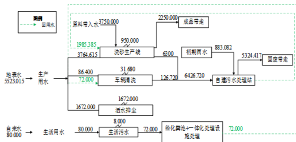
图2-1项目雨季全厂水平衡图 (单位: m³/a)
