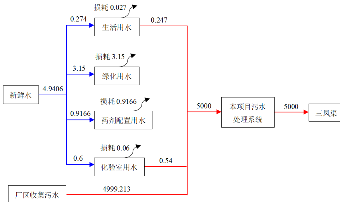
图 3.1-5 项目晴天用水一览表 单位：m 3 /d
