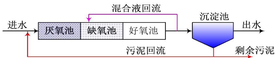
图 3.2-2 AAO 工艺基本流程
