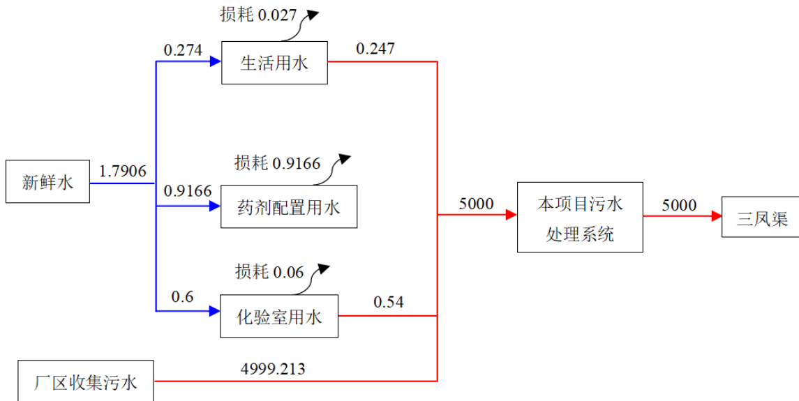
图 3.1-6 项目雨天用水一览表 单位: \text{m}^3/\text{d}
