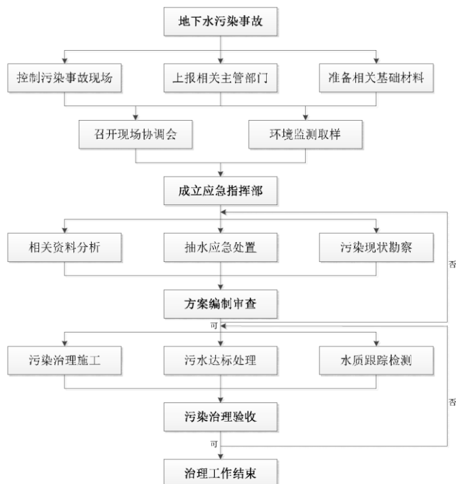
图 5.5-2 地下水污染应急治理程序
