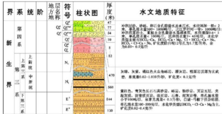
综合水文地质柱状剖面图
