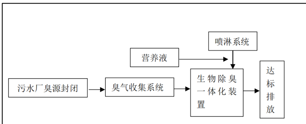
图 6.3-1 项目废气治理工艺流程图
