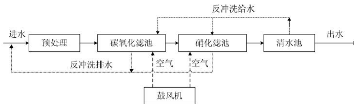
图 3.2-8 碳氧化滤池+硝化滤池两级组合工艺流程图
