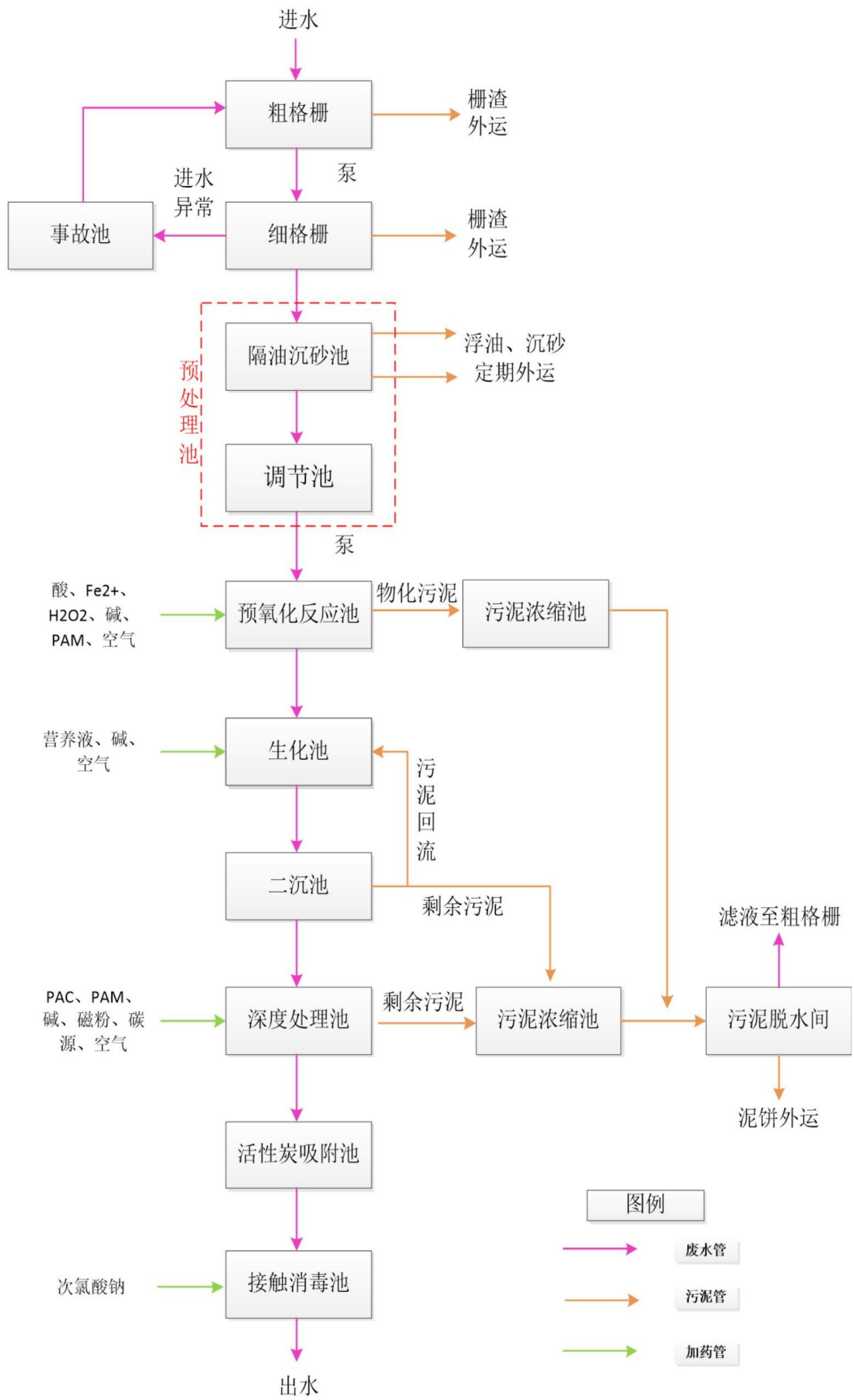
图 6.2-1 污水处理工程工艺流程图
